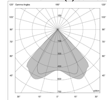
WIDE OPTIC (D) 60°X 90°
